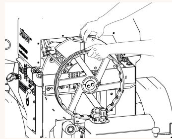
Abbildung 51 - Die Hackscheibe zu sich ziehen
