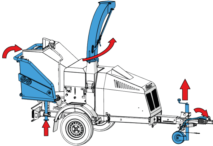
Abbildung 24 - Transportstellung
