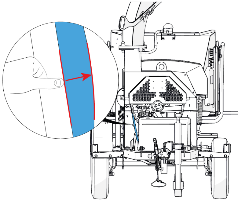
Abbildung 65 - Korrekte Spannung der Hauptkeilriemen
