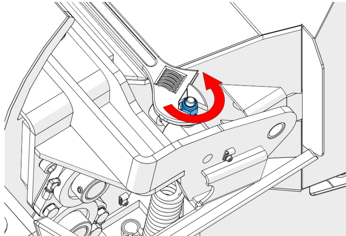
Abbildung 41 - Aufhänger
