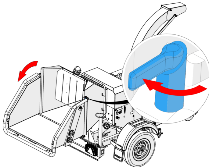
Abbildung 31 - Einzugstisch verriegelt
