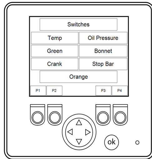
Abbildung 13 - Sensorstatus-Bildschirm
