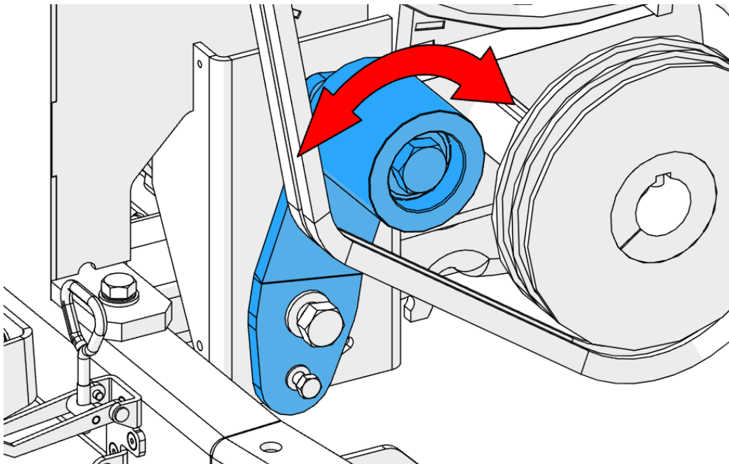
Abbildung 66 - Spannung einstellen
