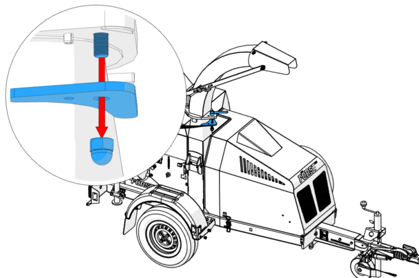
Abbildung 27 - Klemmplatte entfernen
