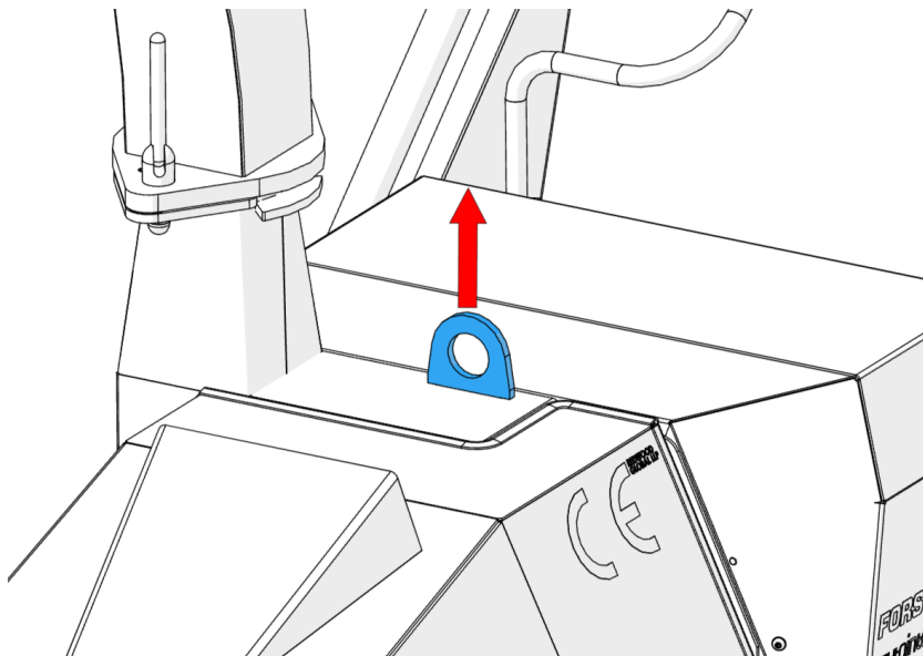
Abbildung 25 - Hebeöse
