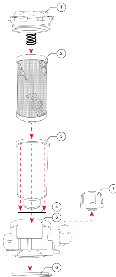
Abbildung 67 - Hydraulikölfilter
