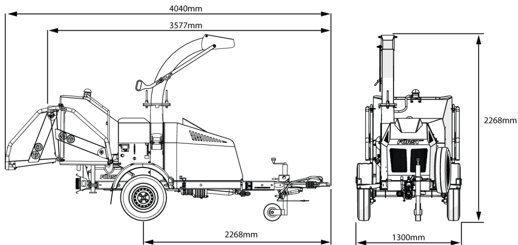
Abbildung 2 - Maße
