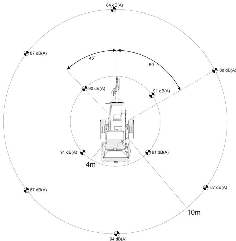
Abbildung 19 - Testergebnisse
