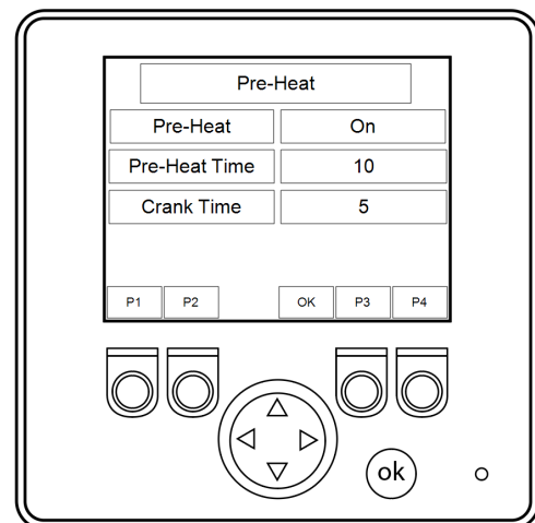
Abbildung 12 - Vorheizsieb
