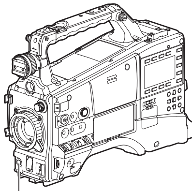
<REC> button
